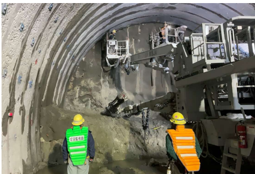
発破掘削 爆薬の装填状況 (広瀬工区)
