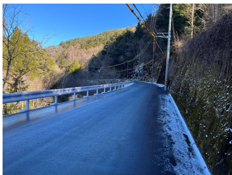
村道区間② 舗装工、ガードレール工 2026年1月7日
