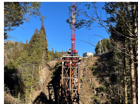
う回路 仮橋工 2026年1月7日
