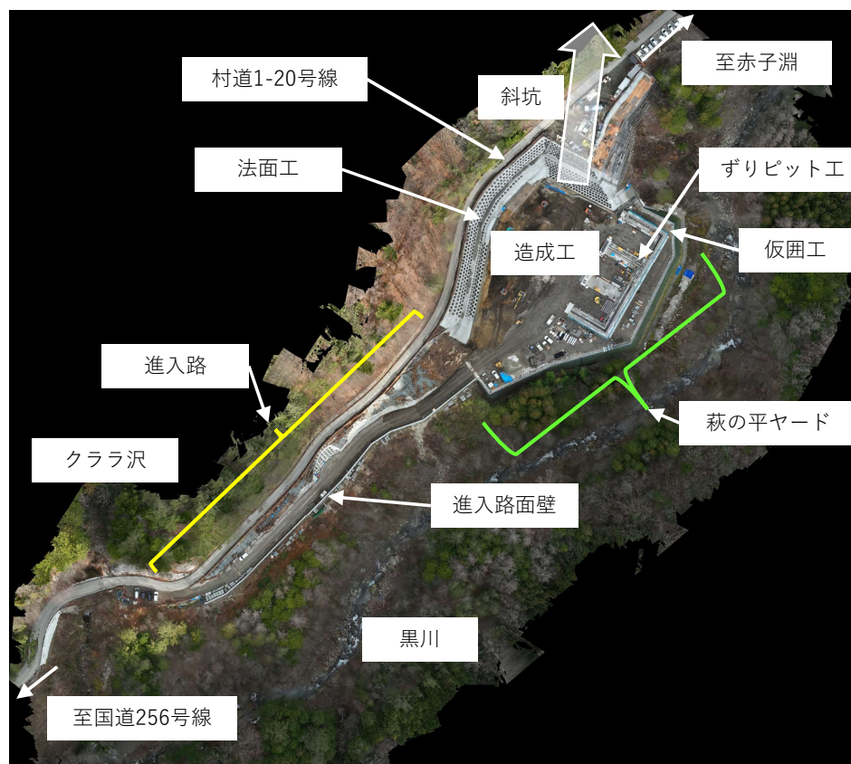
非常口ヤード, 進入路 ドローン撮影 2025年12月17日
