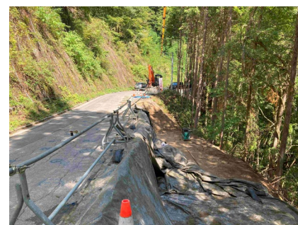
村道区間③ L型擁壁工 2025年10月2日
