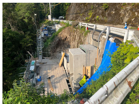
村道区間②池の洞 BOX擁壁工 2025年7月30日
