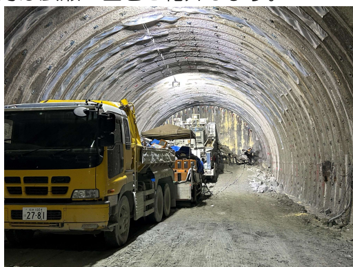
斜坑_補助工法(AGF)施工状況
