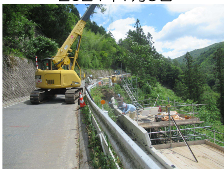
村道区間⑤ パンウォール工_パネル設置 2024年7月9日
