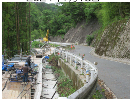
村道区間⑤ さっこう パンウォール工_削孔 2024年7月2日
