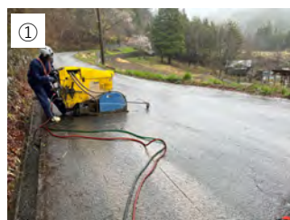
① 【カッター切断】 舗装をカッターで切断します。
