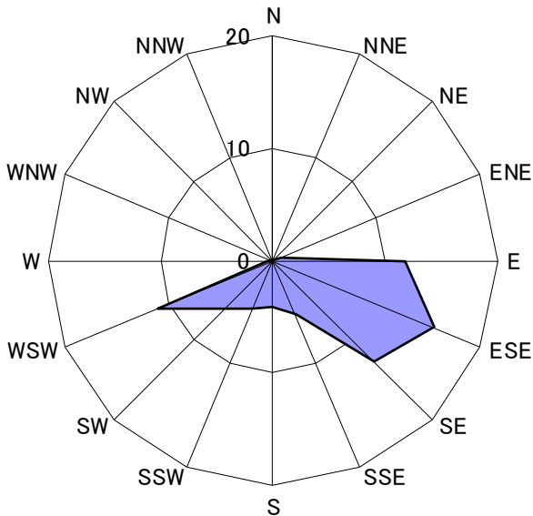
風配図
